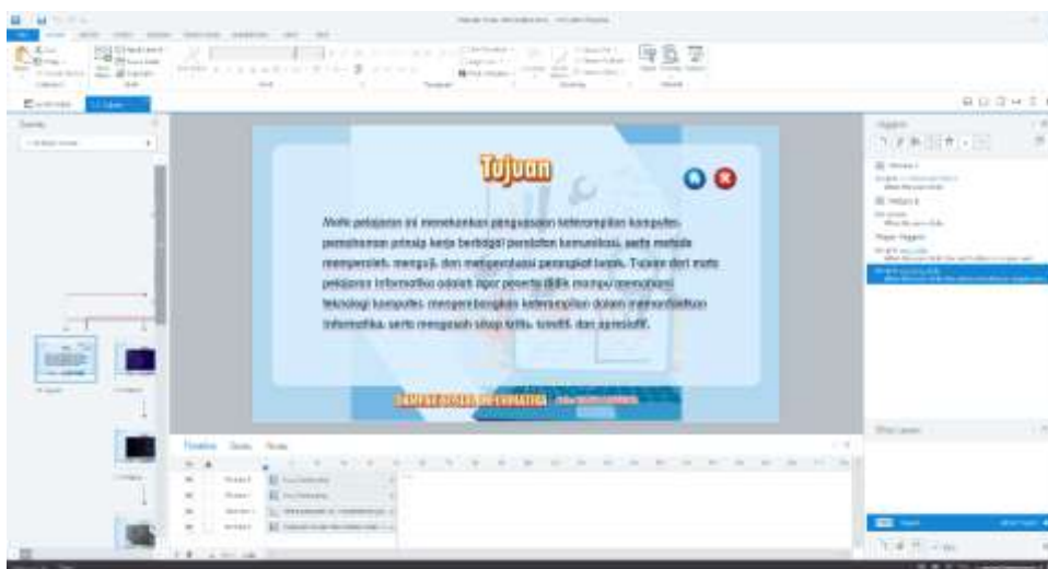
Gambar 4 Halaman Tujuan
